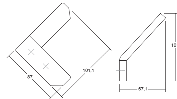
Fixation with screws Fijación con tornillos
